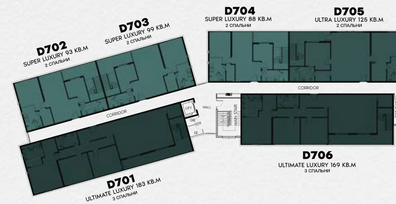
7ой ЭТАЖ
